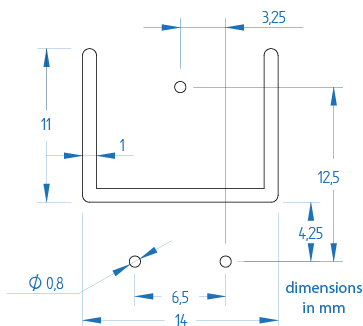
PCB Template
